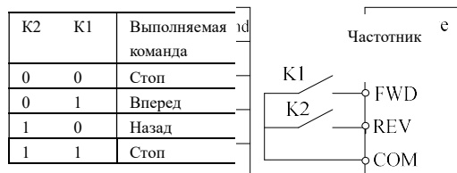
Рис.6-13 Двухпроводной режим управления 1
