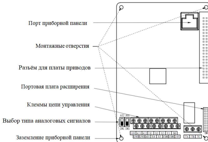
Рис. 3-16 Плата управления
