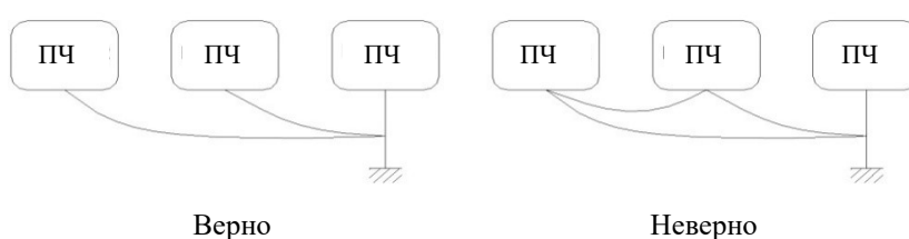
Рис. 3-5 Заземление
