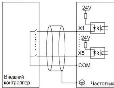
Рис. 3-10 Схема подключения цепи управления
